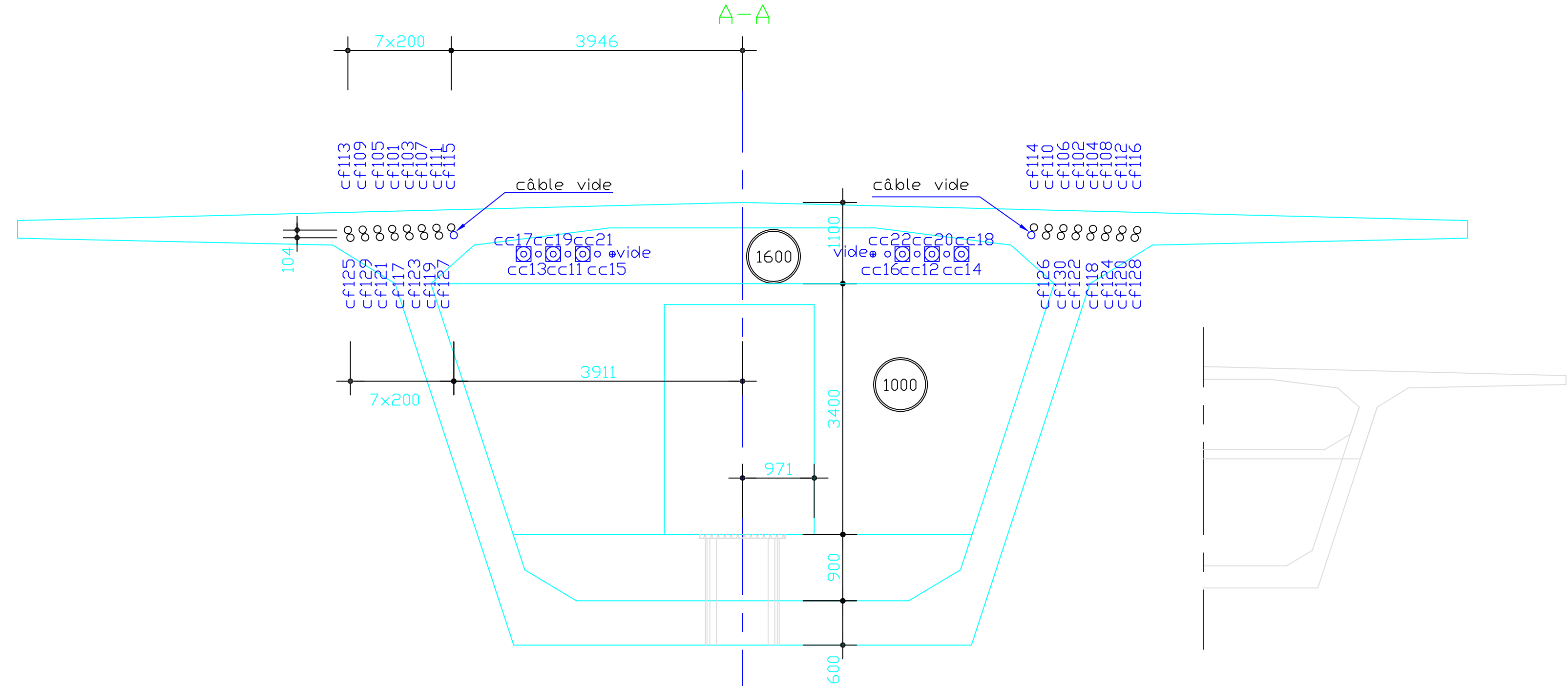
Coupe transversale sur pile (VSP P2 et P3)
