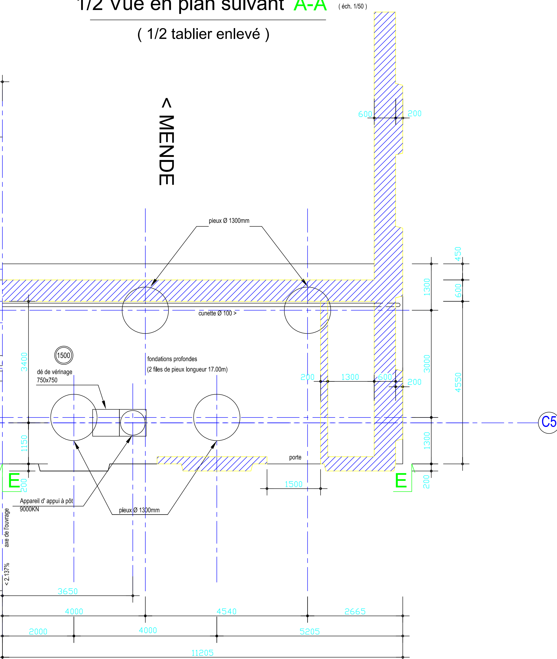
1/2 Vue en plan suivant A-A (éch. 1/50)
