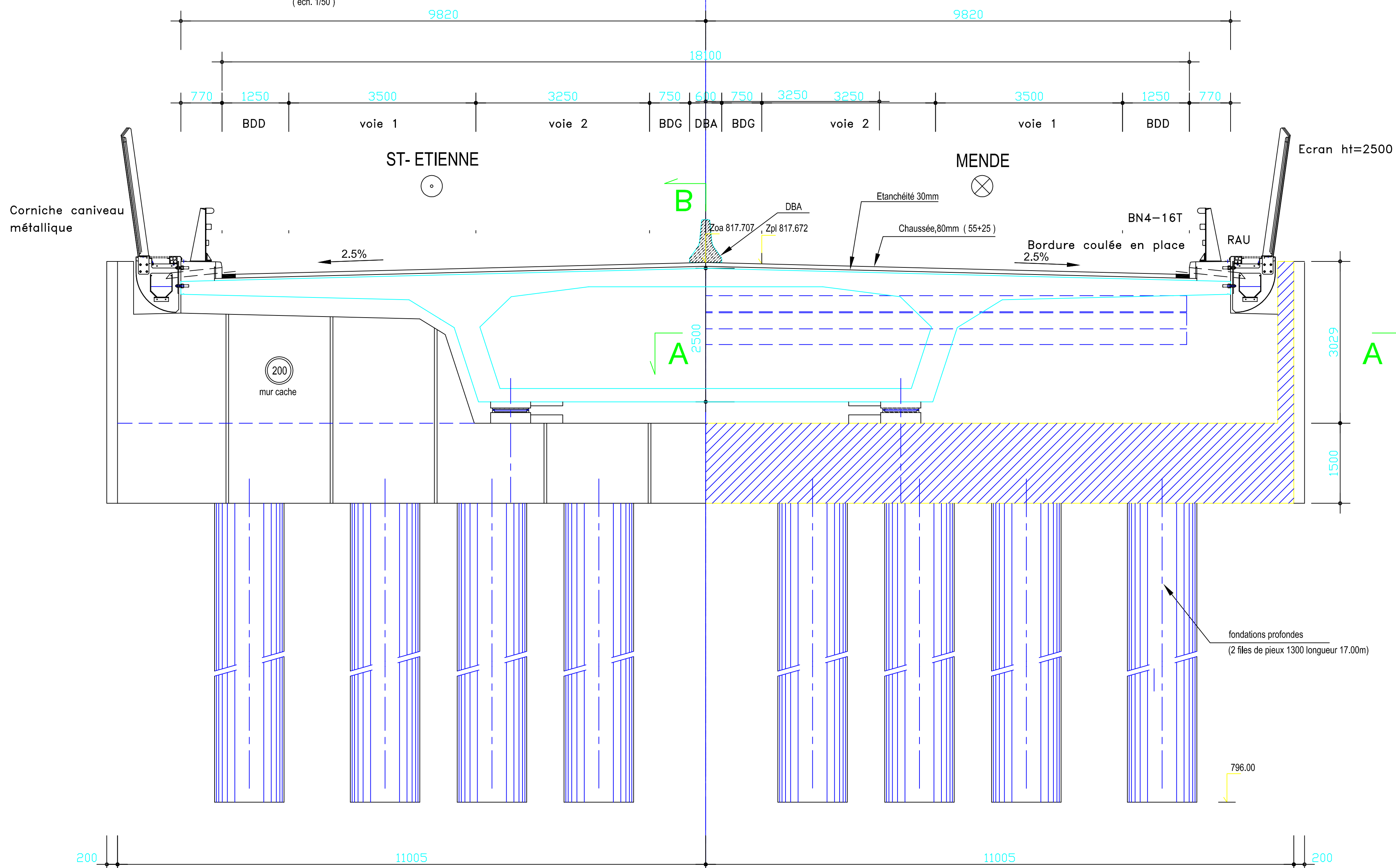
1/2 élévation face avant de la culée C0
